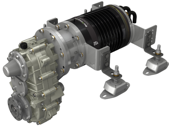
TorqueMaster
